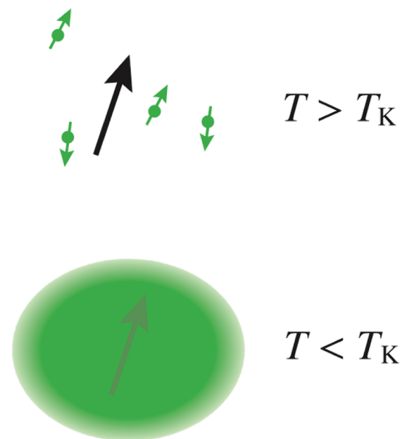
図：近藤効果の概念図。上図は近藤温度 T_K より高温の状態で伝導電子（緑矢印）と不純物スピン（黒矢印）は独立に振る舞う。下図は低温状態で、不純物スピンは伝導電子スピンにより遮蔽される。
